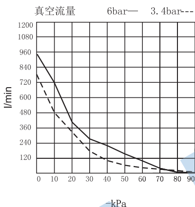
不同真空度 (-kPa) 的真空流量 (l/min)
