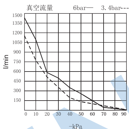
不同真空度 (-kPa) 的真空流量 (l/min)
